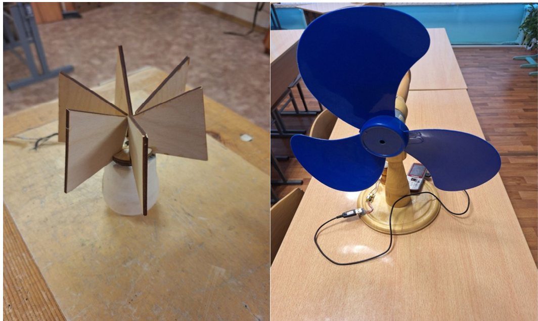
Рис. 7. Вертикальный и горизонтальный ветрогенераторы
