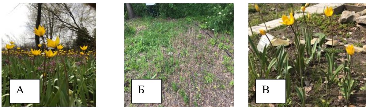
Рисунок 3. Фенология T. biebersteiniana в Пензенском ботаническом саду (А – микрораспуляция 2 «Большая поляна» 30 апреля 2021 г., Б – то же 3 июня 2021 г.; В – микрораспуляция 1 на участке редких растений Природной флоры; 6 мая 2021 г.)
