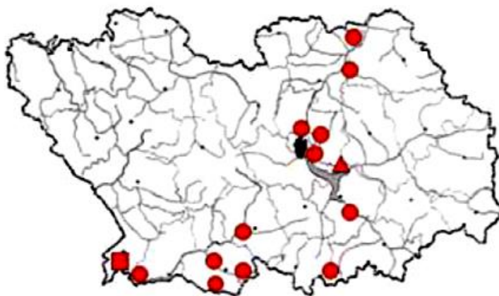
Рисунок 1. Распространение T. biebersteiniana в Пензенской области [Красная Книга Пензенской области т.1]
